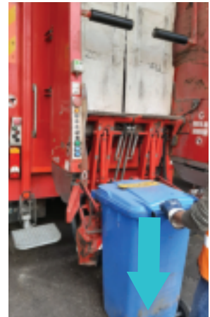
Descente du bac vide
